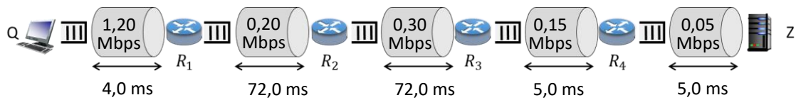
Abbildung 1: Übertragungsstrecke
